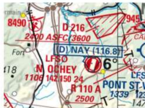
Exemple de représentation sur la carte OACI-VFR :
